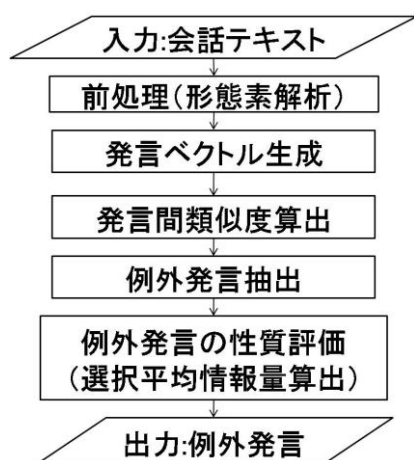
図 2 テキスト処理フローチャート
